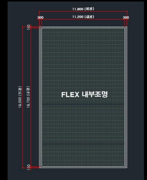
< 외경/내경 참고 도면 >
